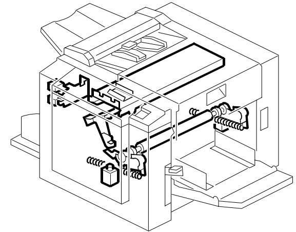
9. PRESS ROLLER SECTION (C261)
