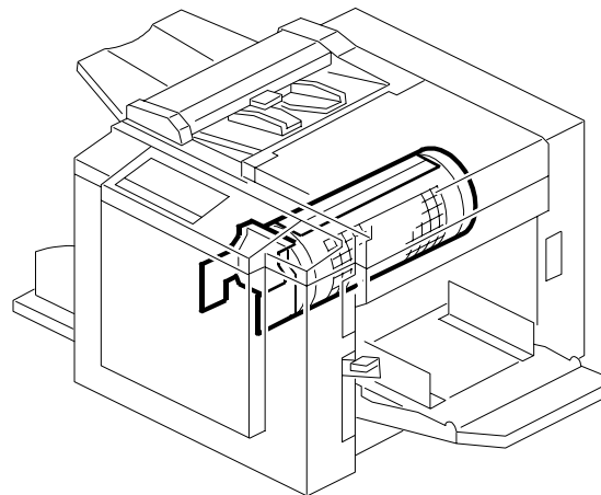
11. DRUM UNIT 2 (C261)
