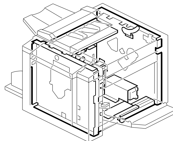
18. FRAME SECTION (C252)
