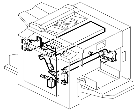
9. PRESS ROLLER SECTION (C252)
