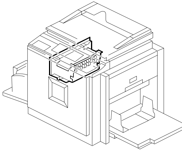
20. Master Eject Unit 1 (C264)
