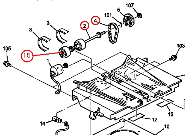
16.Vacuume Fan Unit (C237)
