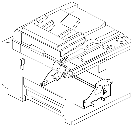
20. Duplex Unit 4 (C269)
