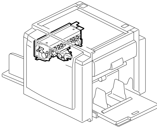
19. MASTER EJECT UNIT 1 (C267)
