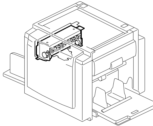
20. MASTER EJECT UNIT 2 (C267)
