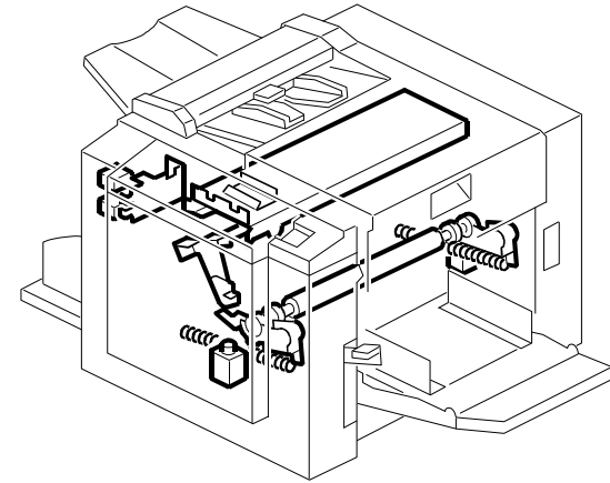
9. Press Roller Section (C274)
