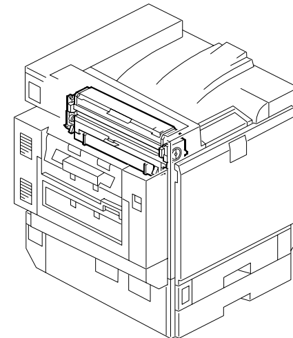
21. Fusing Unit 1 (G130/G131)
