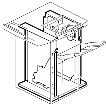
27. Frame Section 2 (D707)
