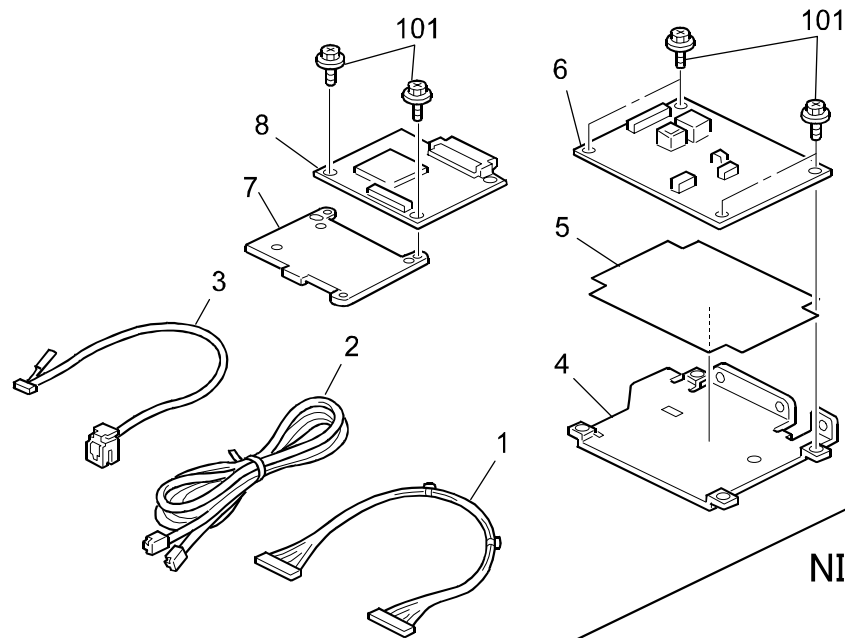
G3 Interface Unit
