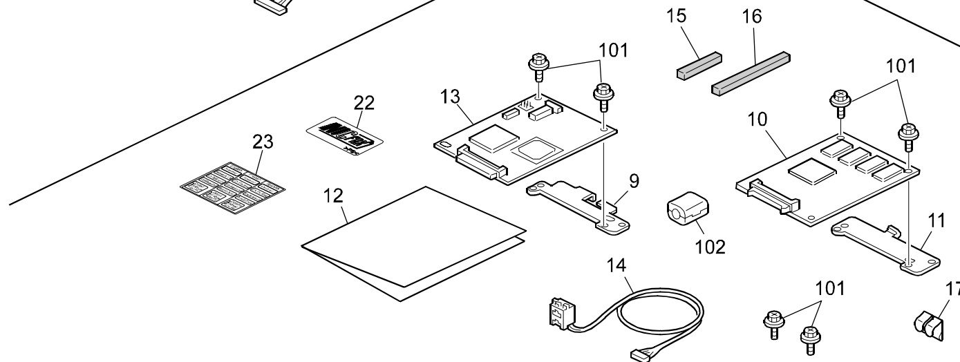
NIC FAX Unit
