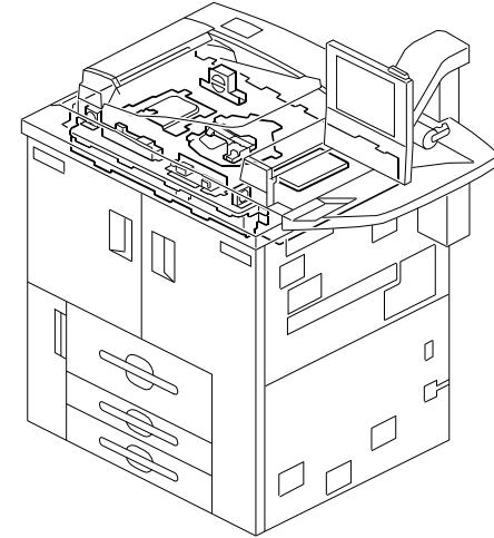
21. Optics Section 3 (D059/D060/D061)
