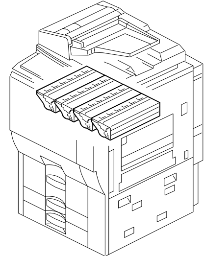
36. PCU 3 (D014/D015)
