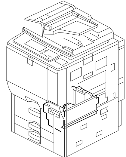
24. Tandem Tray 2 (D014/D015)
