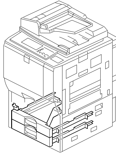
26. Universal Tray 1 (D014/D015)
