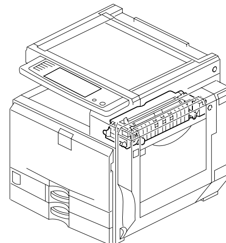
30. Fusing unit 2 (B222/B224)
