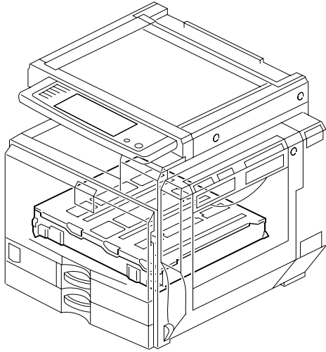
19. LD unit (B222/B224)
