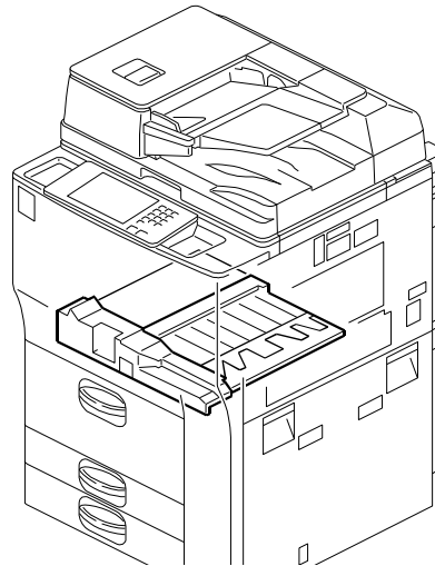
53. Duplex Unit 1 (D131/D132/D133)
