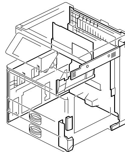
3. Exterior 3 (D182/D183/D184)
