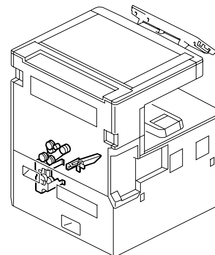
27. Drive Section 2 (D182/D183/D184)
