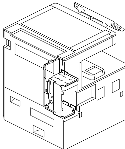
29. Electrical Section 1 (D182/D183/D184)
