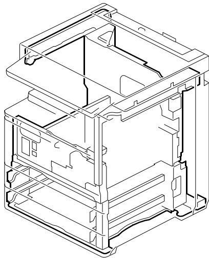
34. Frame Section (D120/D121/D122/D139/D140/D141)
