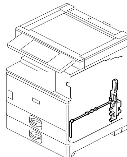
24. Duplex Section 4 (D120/D121/D122/D139/D140/D141)
