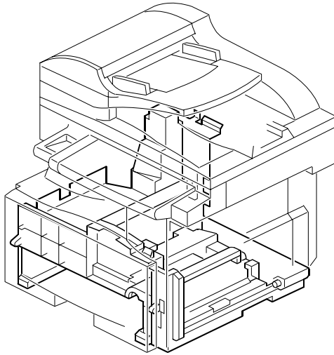
19. Frame Section (B284/B288)
