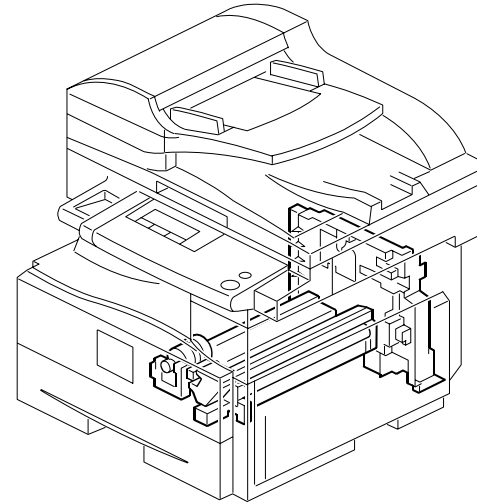
15. PCU Section (B284/B288)
