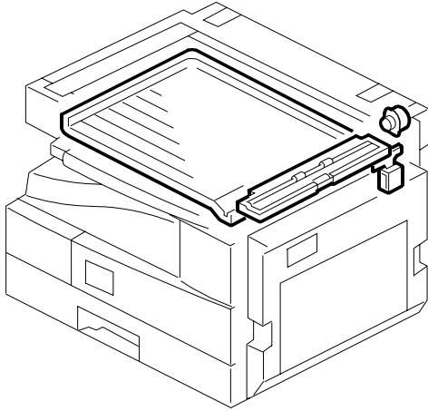
19. Duplex Unit 3 (B282-62)
