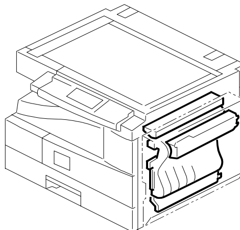
17. Duplex Unit 1 (B282)
