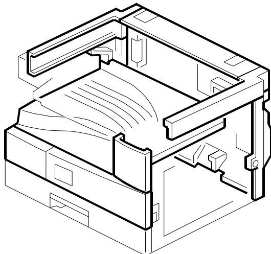
1. Exterior 1 (B282/B283)
