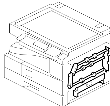
18. Duplex Unit 2 (B282)
