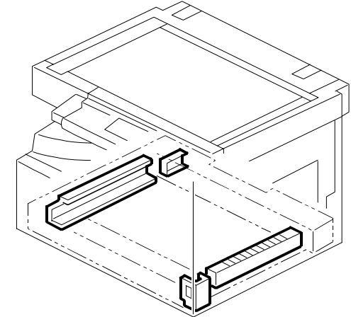
24. Frame Section 2 (B282/B283)
