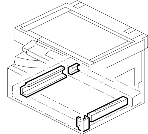
24. FRAME SECTION 2 (B282)
