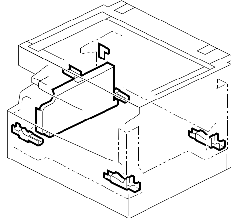
23. FRAME SECTION 1 (B283)
