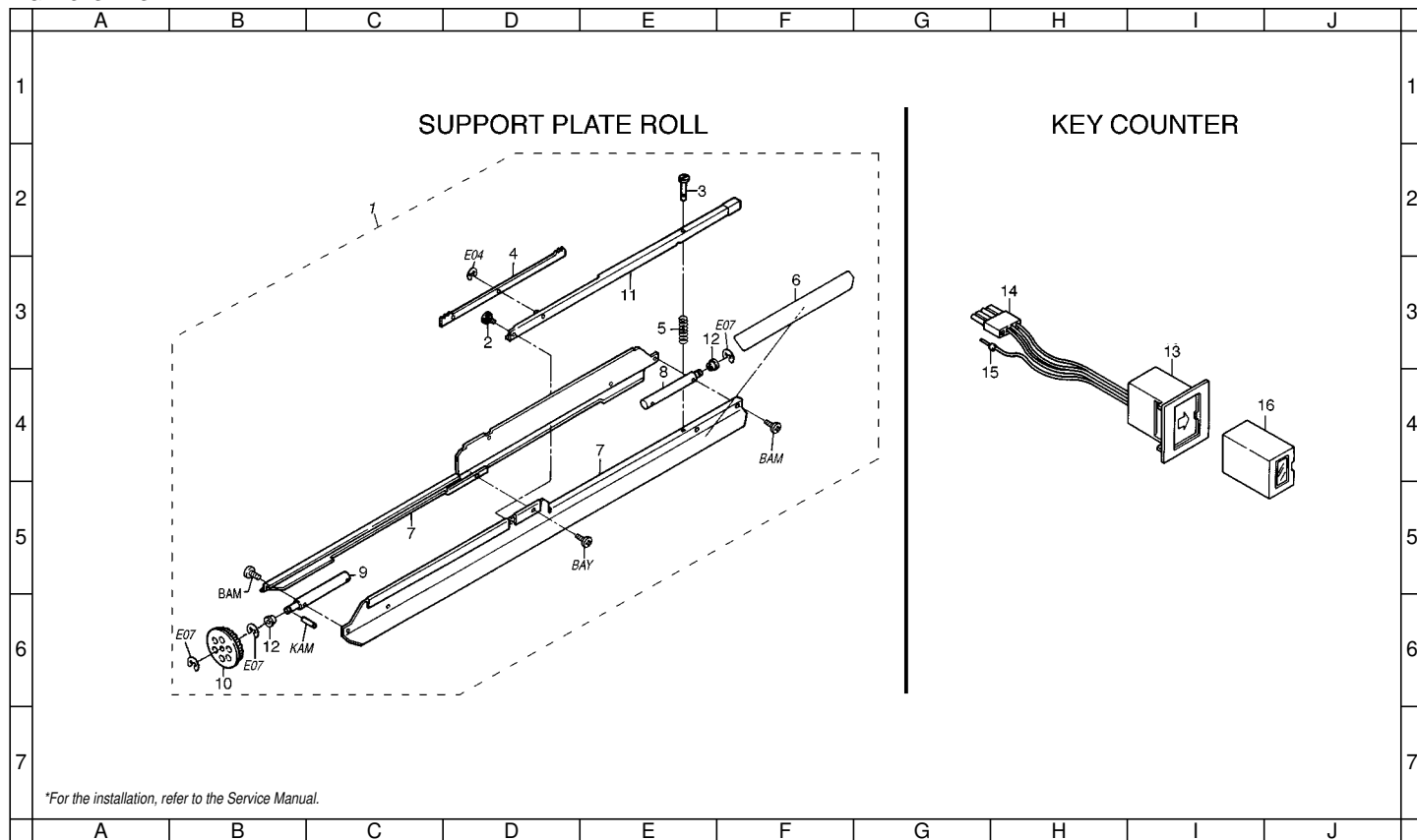
FIG. 23 OPTION 2
