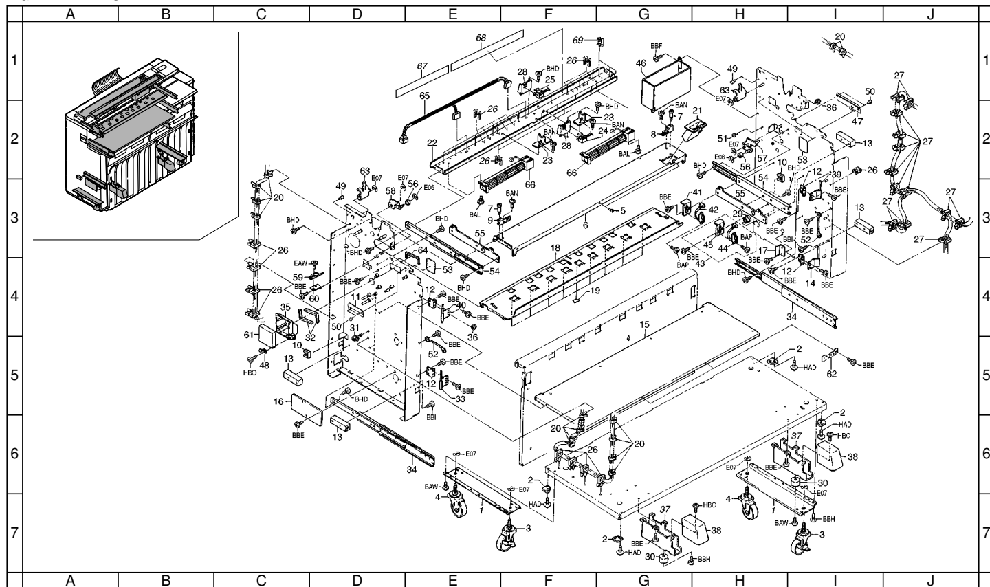
FIG. 2 FRAMES
