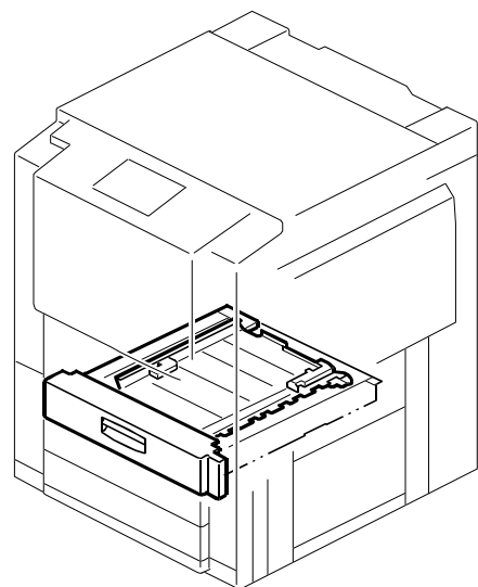
40.DUPLEX UNIT 1 (A257/A269)
