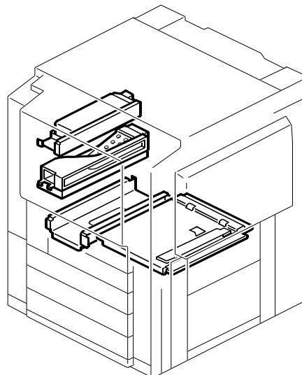
56.FRAME SECTION 2 (A257/A269)
