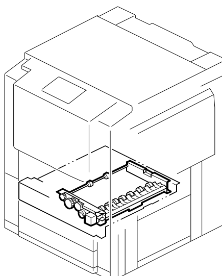
41.DUPLEX UNIT 2 (A257/A269)
