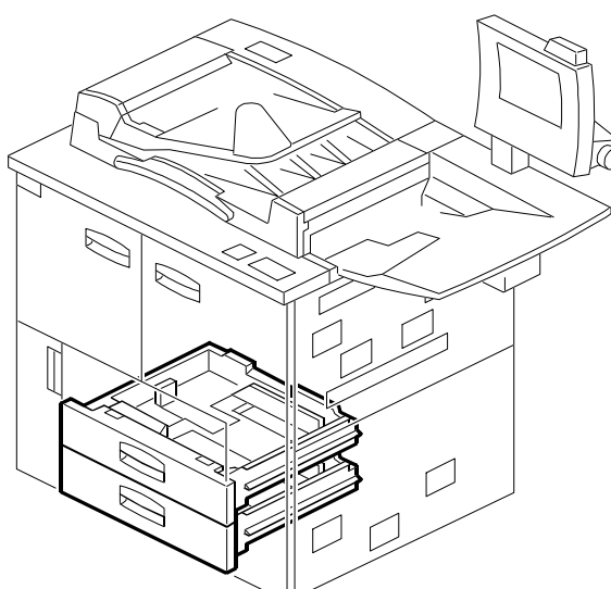
23.UNIVERSAL TRAY (A294)
