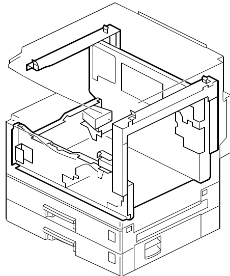
25.FRAME SECTION (A265/A267)
