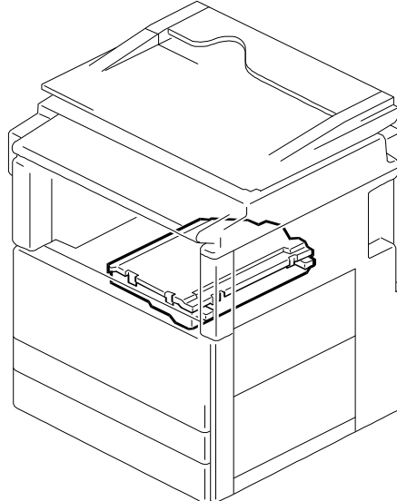
11. Laser Unit (A193)
