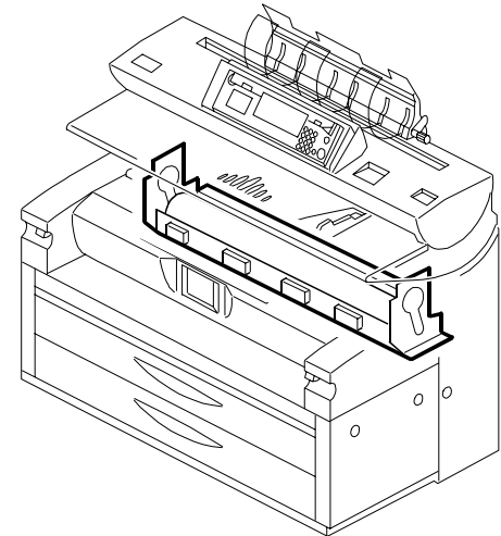
24. FUSING UNIT 2 (B010)
