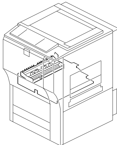
56. Duplex Unit 2 (B132/B181/B200)
