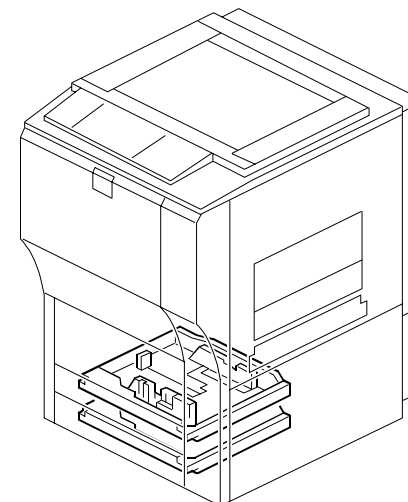
27. Universal Tray 2 (B132/B181/B200)
