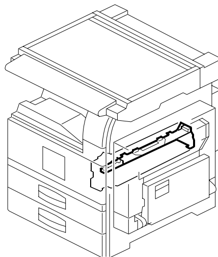
17. OPC UNIT 1 (B195/B198/B264/B265)
