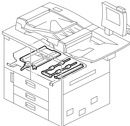
56. DUPLEX UNIT 4 (B070/B071)
