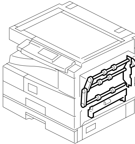
20. DUPLEX UNIT 2 (B123/B261)
